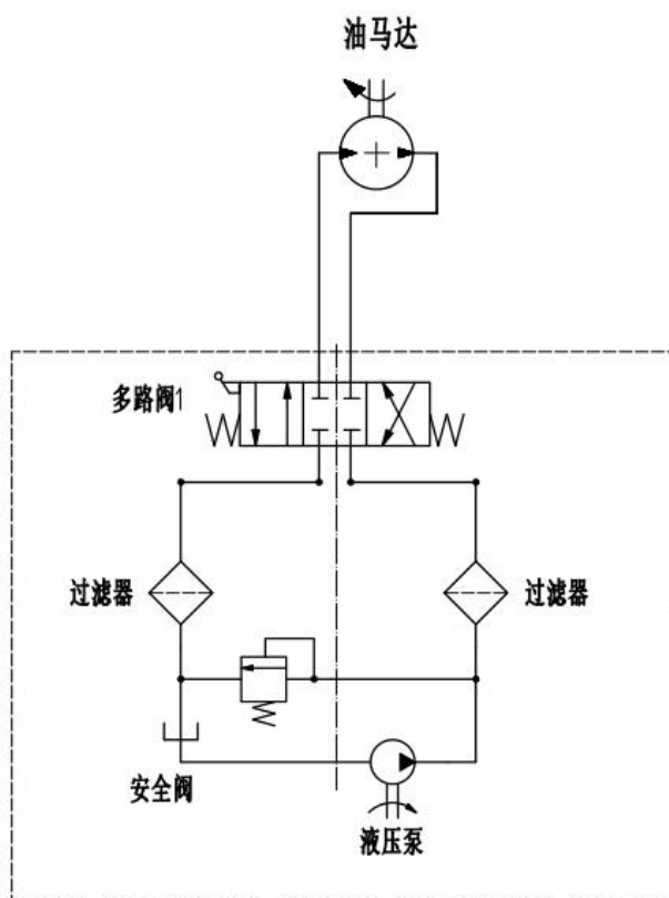
旋转器液压原理图
